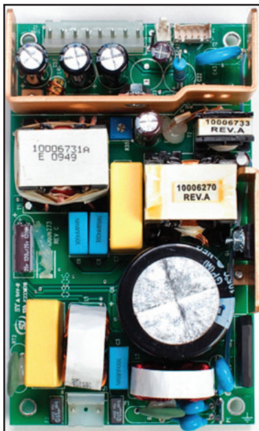
그림 8-6 전원 모듈
