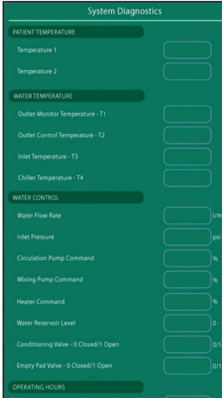
그림 7-1 시스템 진단
