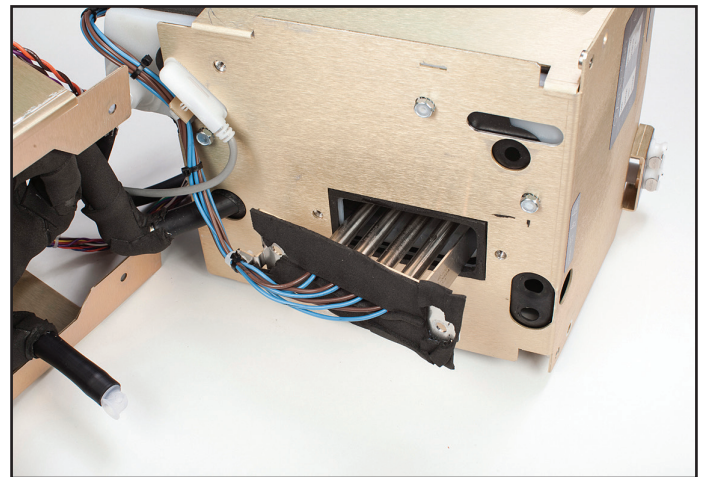
그림 8-50 히터 제거(4단계)
